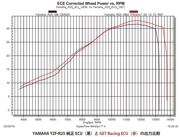
YAMAHA YZF-R25 純正 ECU (黒) と GET Racing ECU (赤) の出力比較
